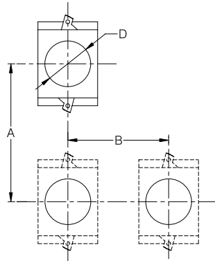
부착간격도
